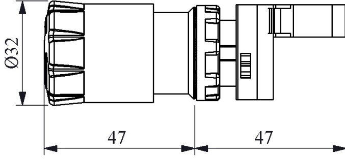
Montaj Ölçüsü \text{Ø}22.4 \pm 0.2 mm
