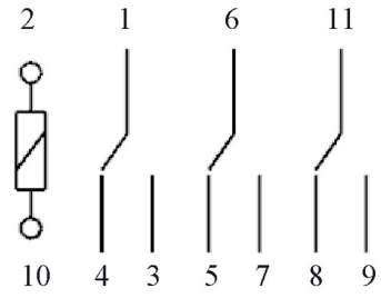
Devre Şeması
