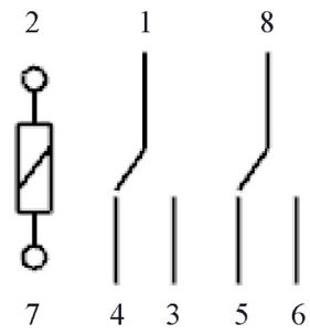
Devre Şeması
