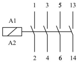
Elektrik Şeması
