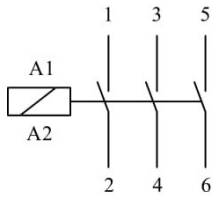
Elektrik Şeması
