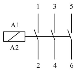
Elektrik Şeması
