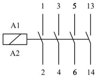
Elektrik Şeması
