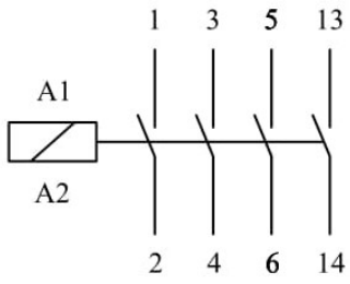
Elektrik Şeması
