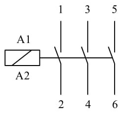
Elektrik Şeması
