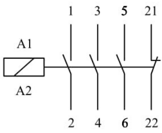
Elektrik Şeması
