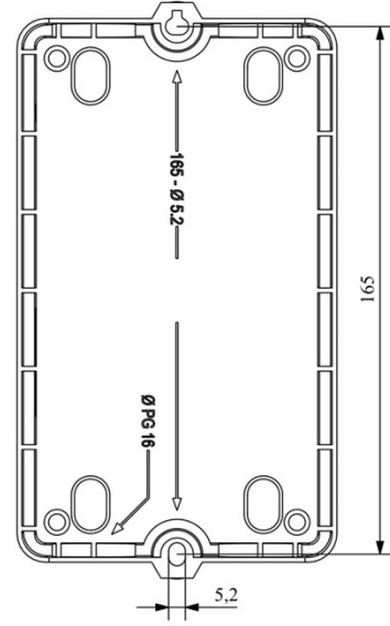
Montaj Ölçüsü
