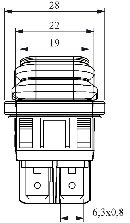
Montaj Ölçüsü 30,2x22,2mm
