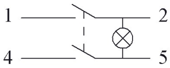
Devre Şeması
